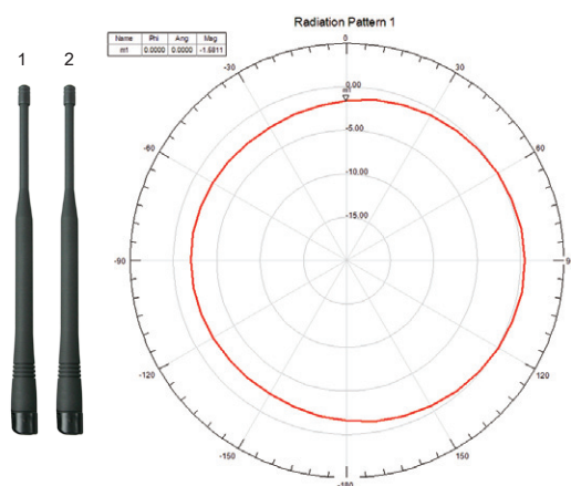
Antenna Pattern (z-axe)
