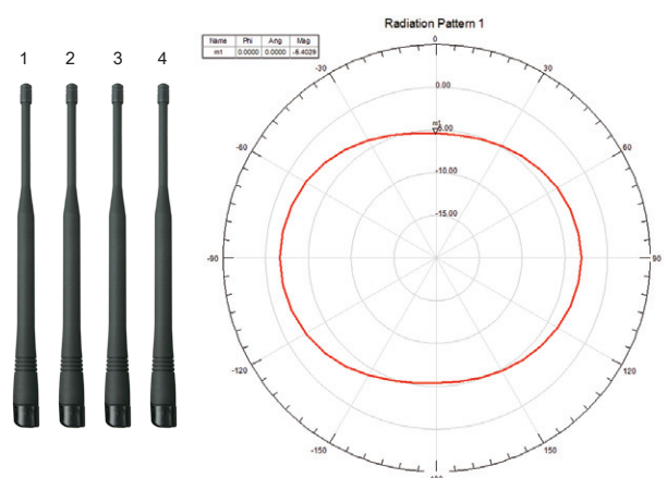
Antenna Pattern (z-axe)
